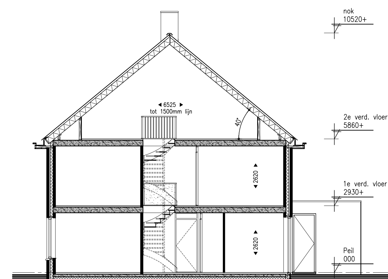
Doorsnede
