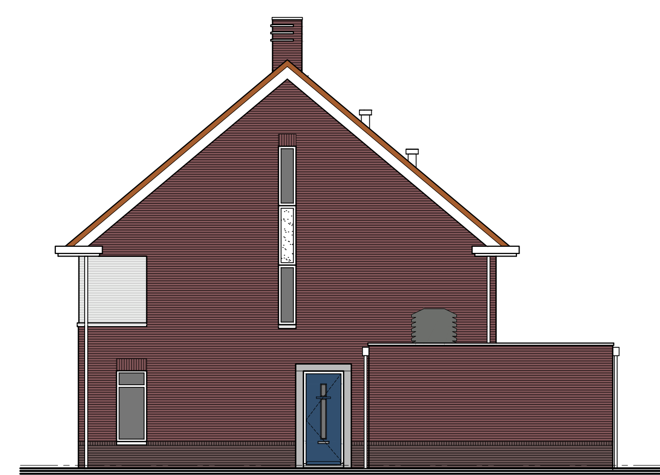
Rechter zijgevel
