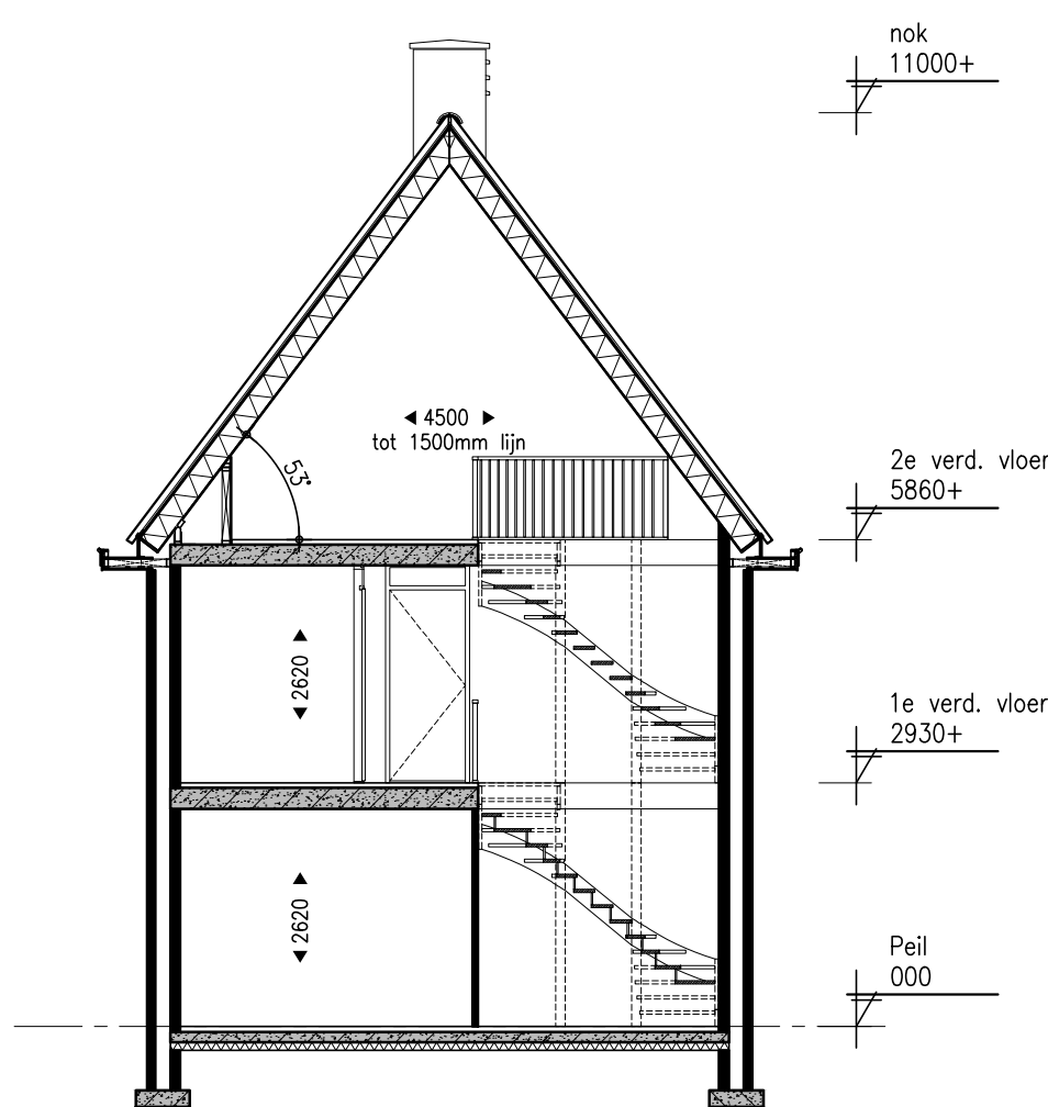
Doorsnede
