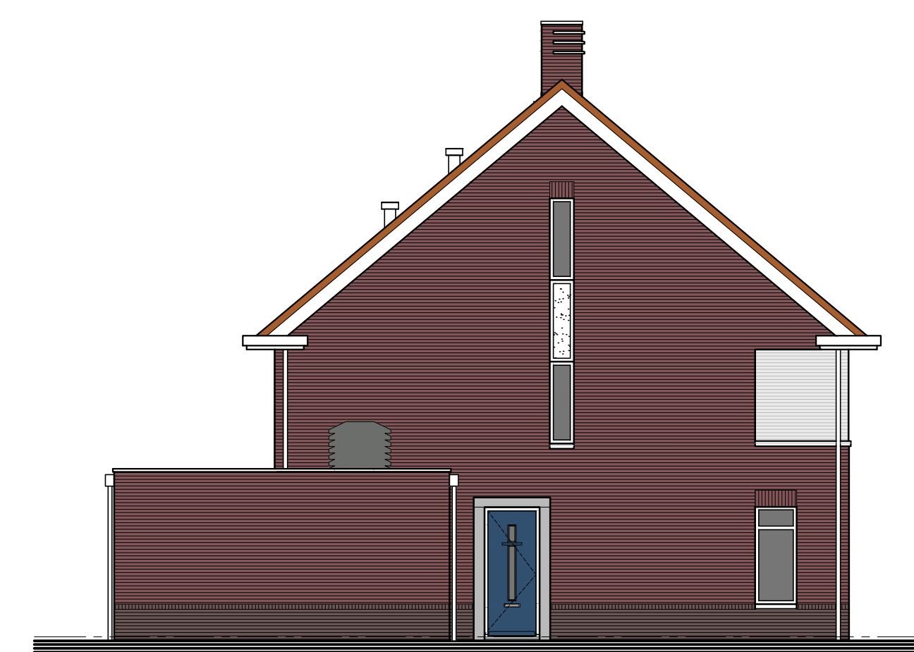
Linker zijgevel
