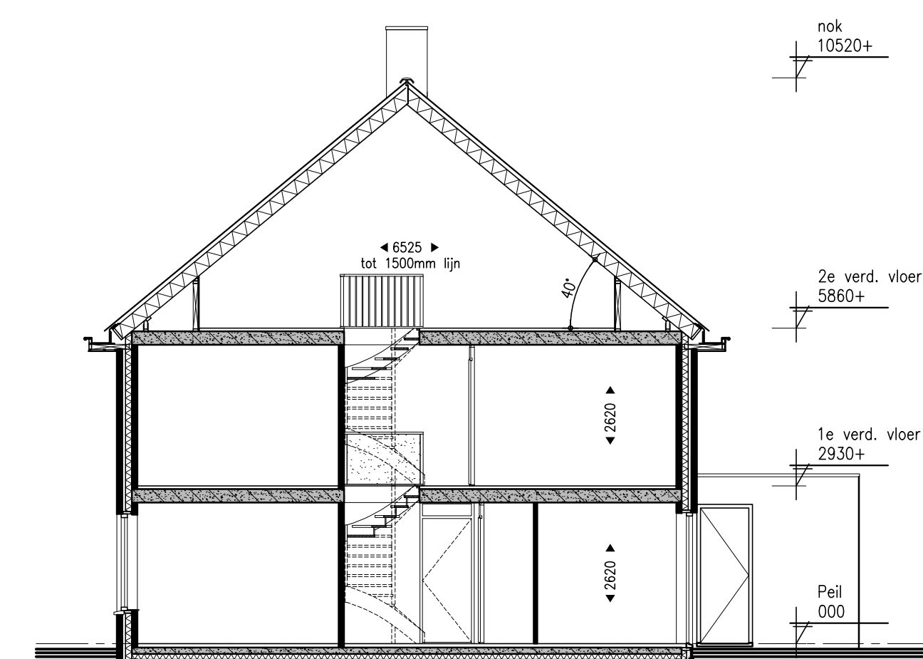
Doorsnede
