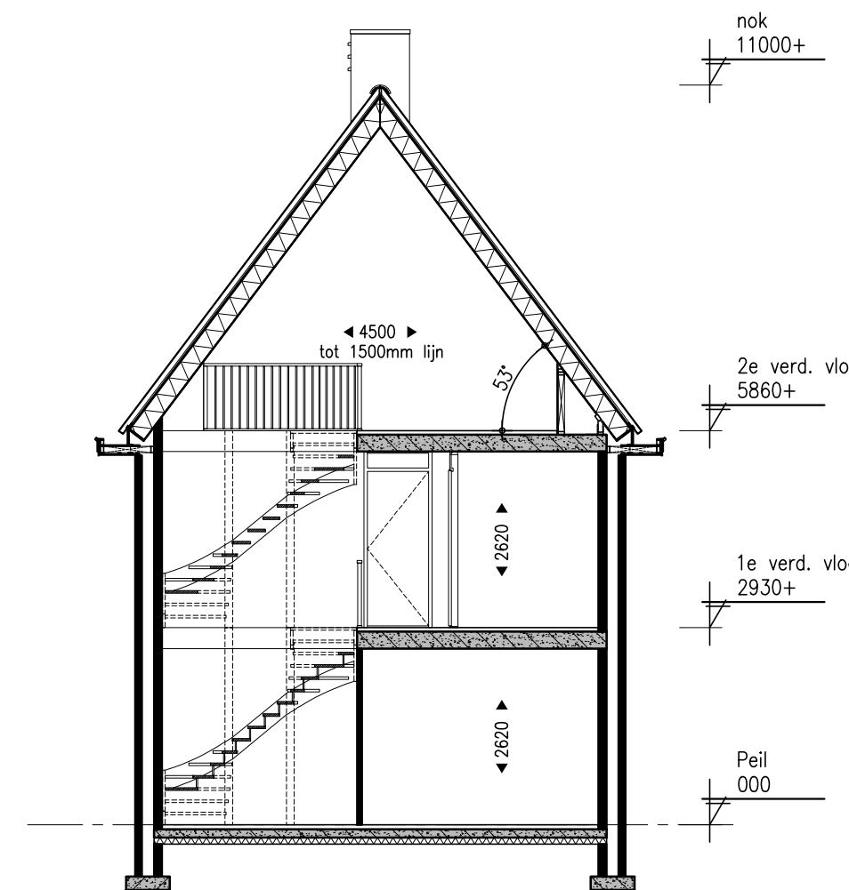
Doorsnede
